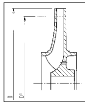
Reduction du diamètre extérieur de la roue pour pompe centrifuge par torneage.
