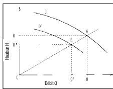
Diagramme pour déterminer le diamètre de torneage.
